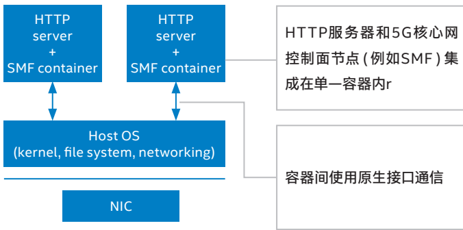
图二 集成式容器SBA架构部署方案
